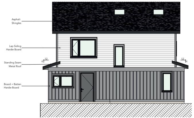
2 D5 North Elevation SCALE: 1/8" = 1'-0"
