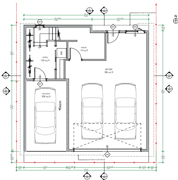
1 D2 Garage Level SCALE: 3/16" = 1'-0"
