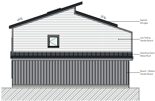
3 D5 West Elevation SCALE: 1/8" = 1'-0"
