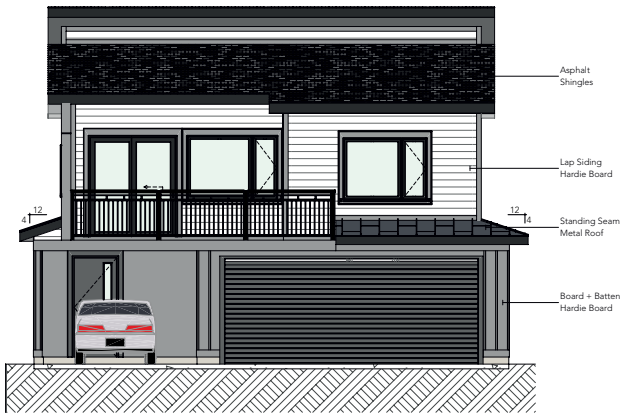
1 D5 South Elevation SCALE: 1/8" = 1'-0"
