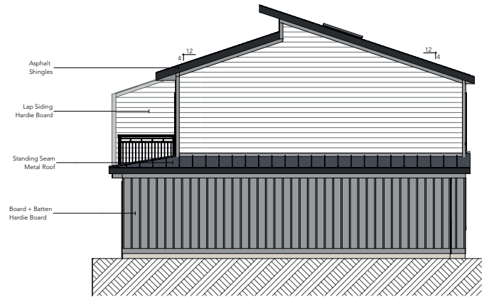
4 D5 East Elevation SCALE: 1/8" = 1'-0"
